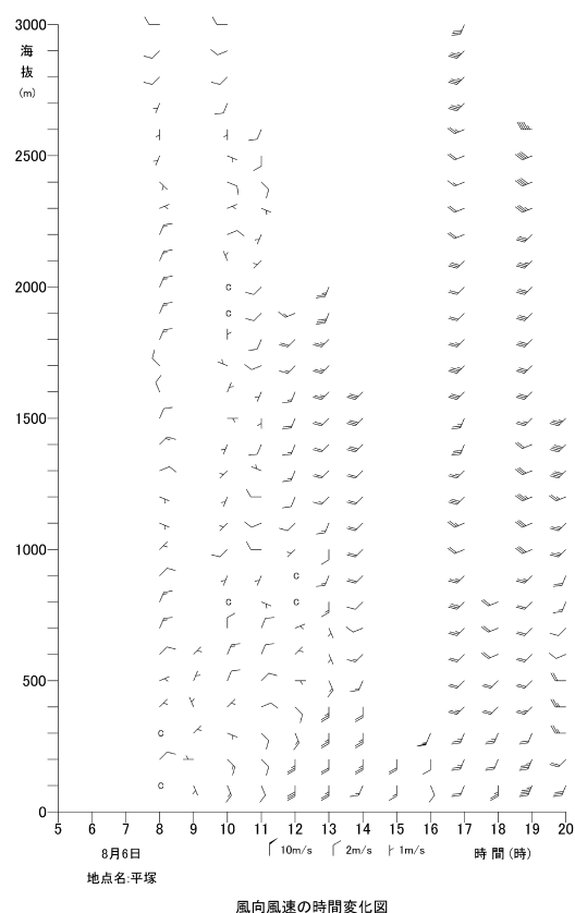
図11 パイロットバルーンによる観測結果
