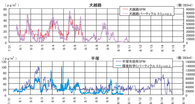
図8 パーティクルカウンタ ( 0.3\mu\text{m} 以上合計) 個数とSPM濃度の比較 (平塚のSPMは常時監視局神田小学校と比較)
