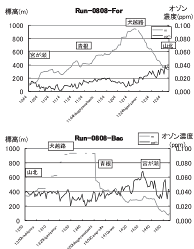
図10 オゾン移動観測の結果 (8/4, 8/5, 8/6 AM, 8/6 PM, 8/8)
