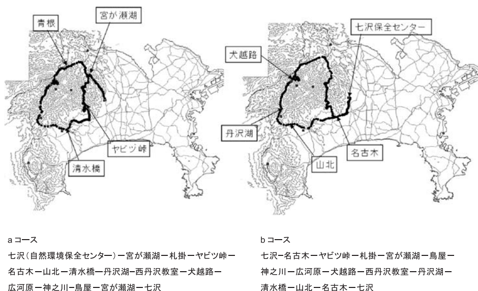
図2 移動車観測をおこなったコース
