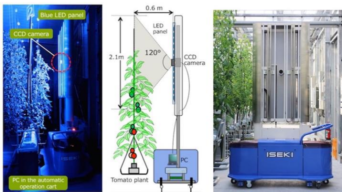
図2 愛媛大学植物工場研究センターの研究成果として井関農機 (株) より市販されたクロロフィル蛍光画像計測ロボット
